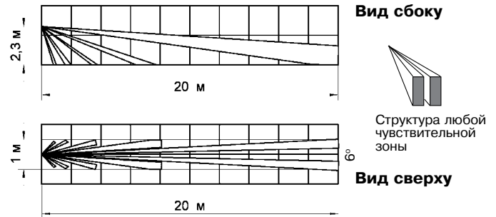
Рисунок 2 – Диаграмма зоны обнаружения
