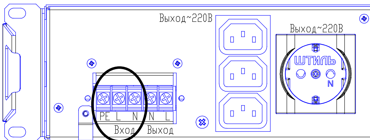
Рисунок 3.2 – Стабилизатор ИнСтаб. Клеммная колодка «Вход РЕ-L-N»
